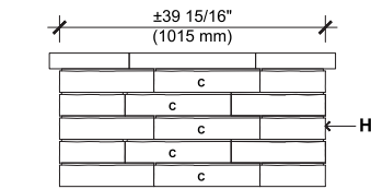
ELEVATION B
