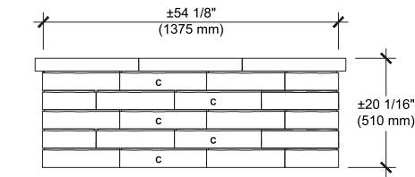
ELEVATION A
