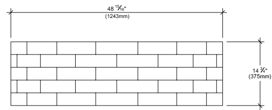
ÉLÉVATION A
