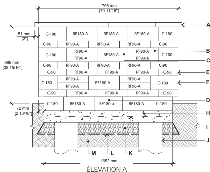
ÉLÉVATION A
