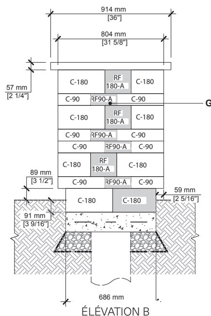
ÉLÉVATION B
