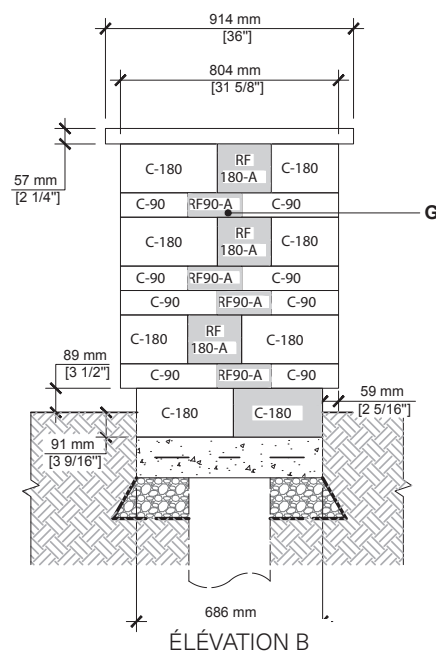
ÉLEVATION B
