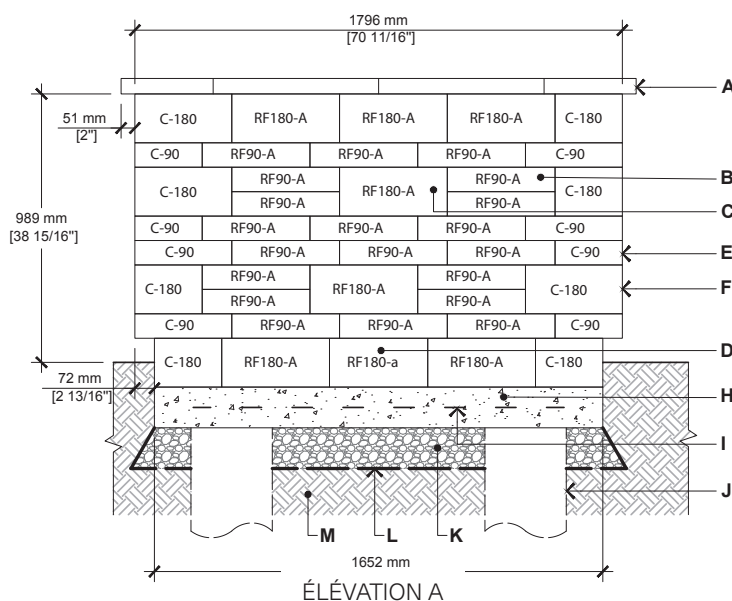
ÉLEVATION A
