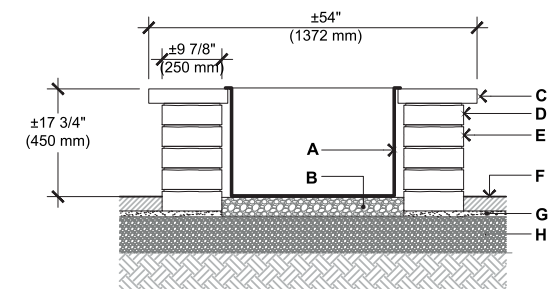
COUPE 1-1
