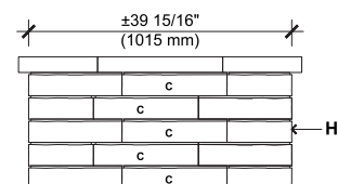
ÉLÉVATION B
