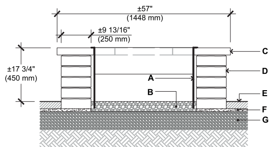
COUPE 1-1
