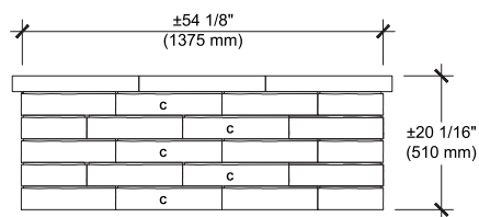
ÉLÉVATION A
