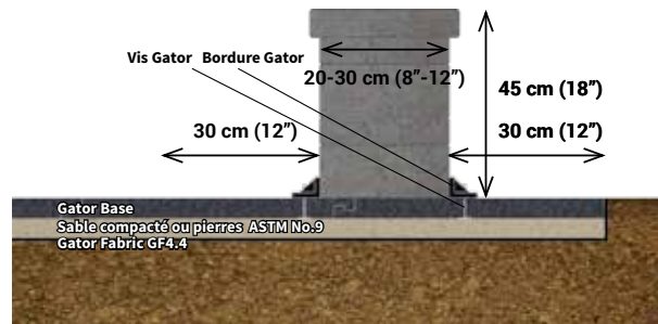
MUR D'ASSISE AUTOPORTANT GRAPHIQUE 6
