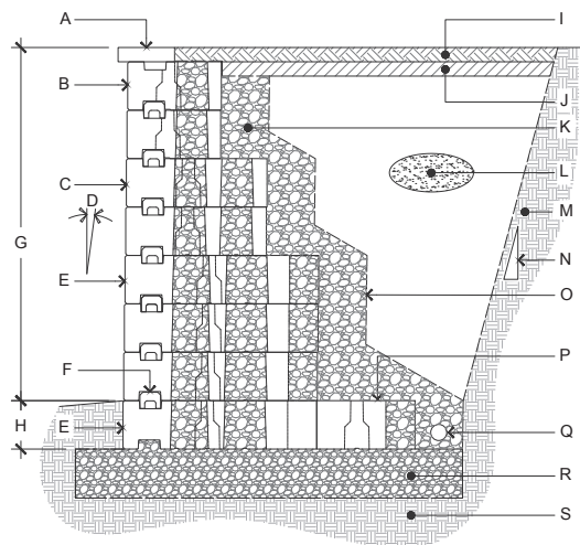
DÉTAIL MUR GRAVITAIRE QUASI-VERTICAL
