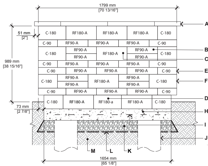
ÉLÉVATION A
