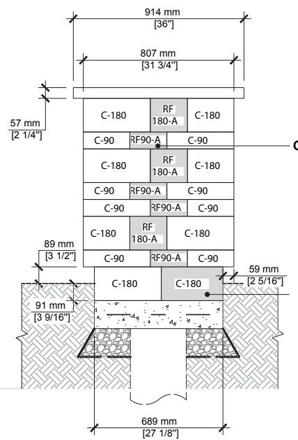
ÉLÉVATION B
