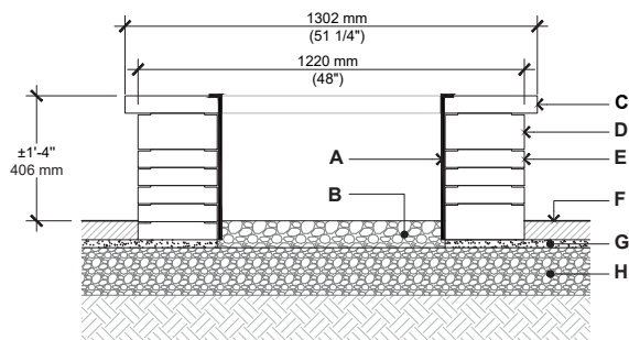
COUPE 1-1
