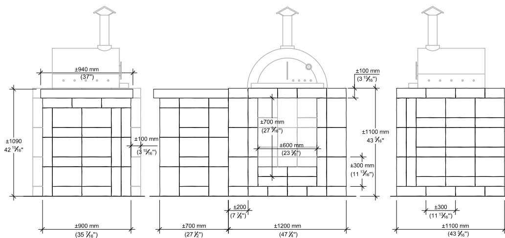
ÉLÉVATION CÔTÉ GAUCHE
