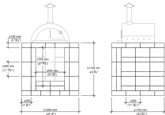
ÉLÉVATION AVANT
