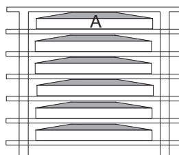
Palette vue de côté - 28" × 28"
