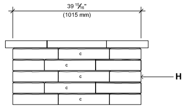
ELEVATION B
